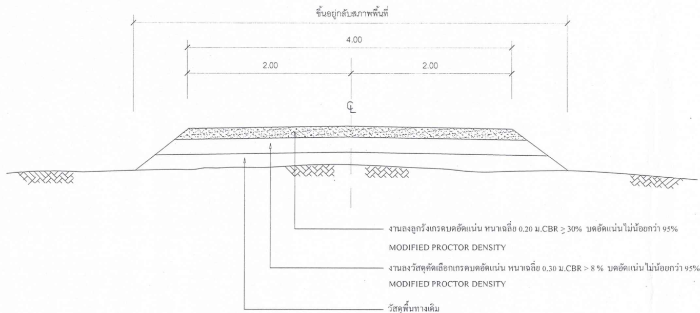
รูปตัดถนนลูกรัง
